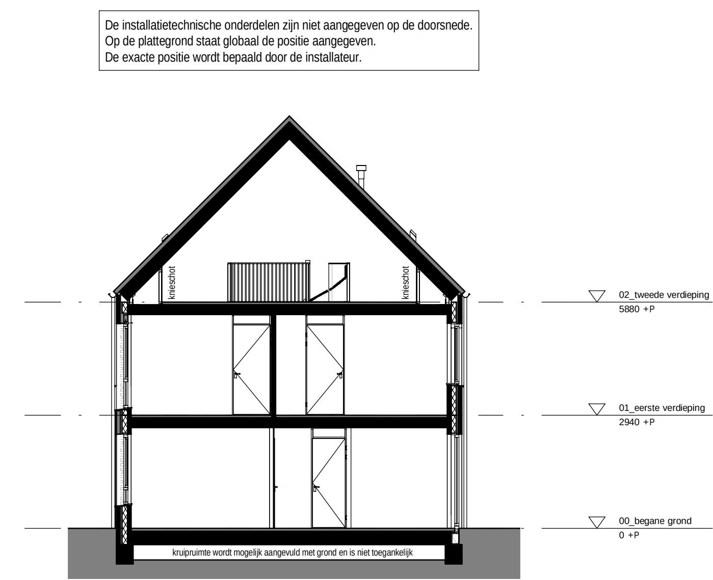
Doorsnede schaal 1:100
