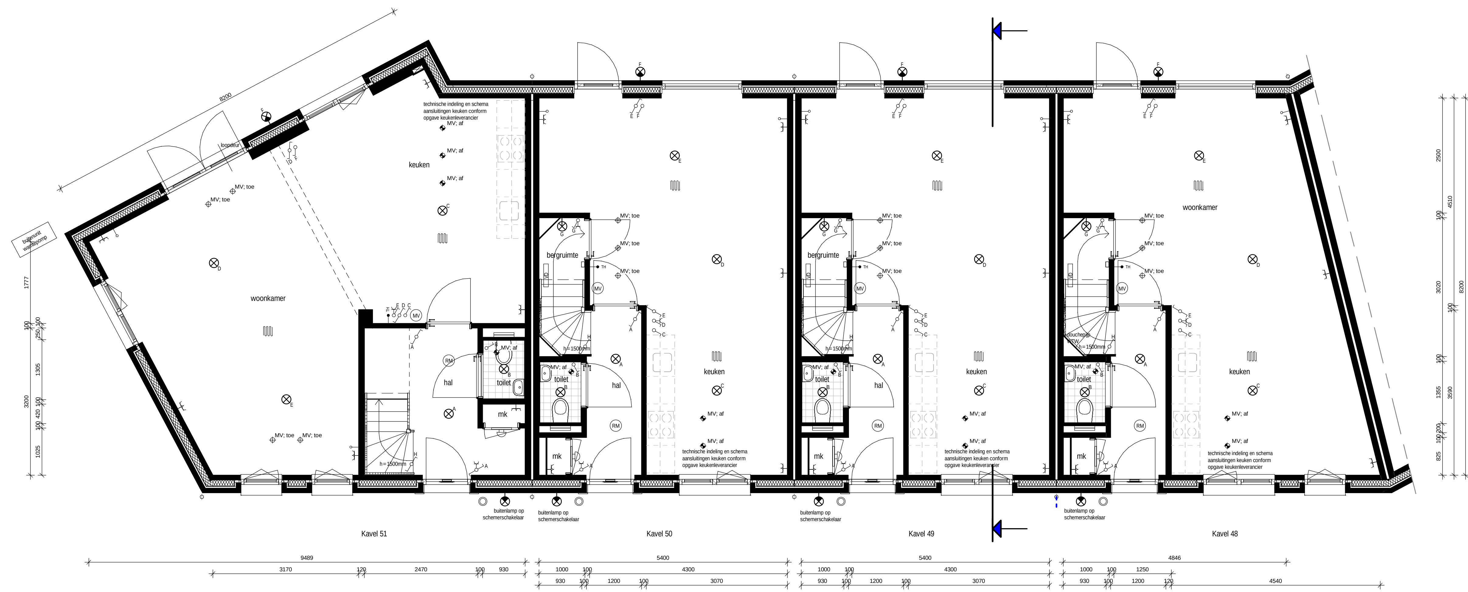
Begane grond schaal 1:50
