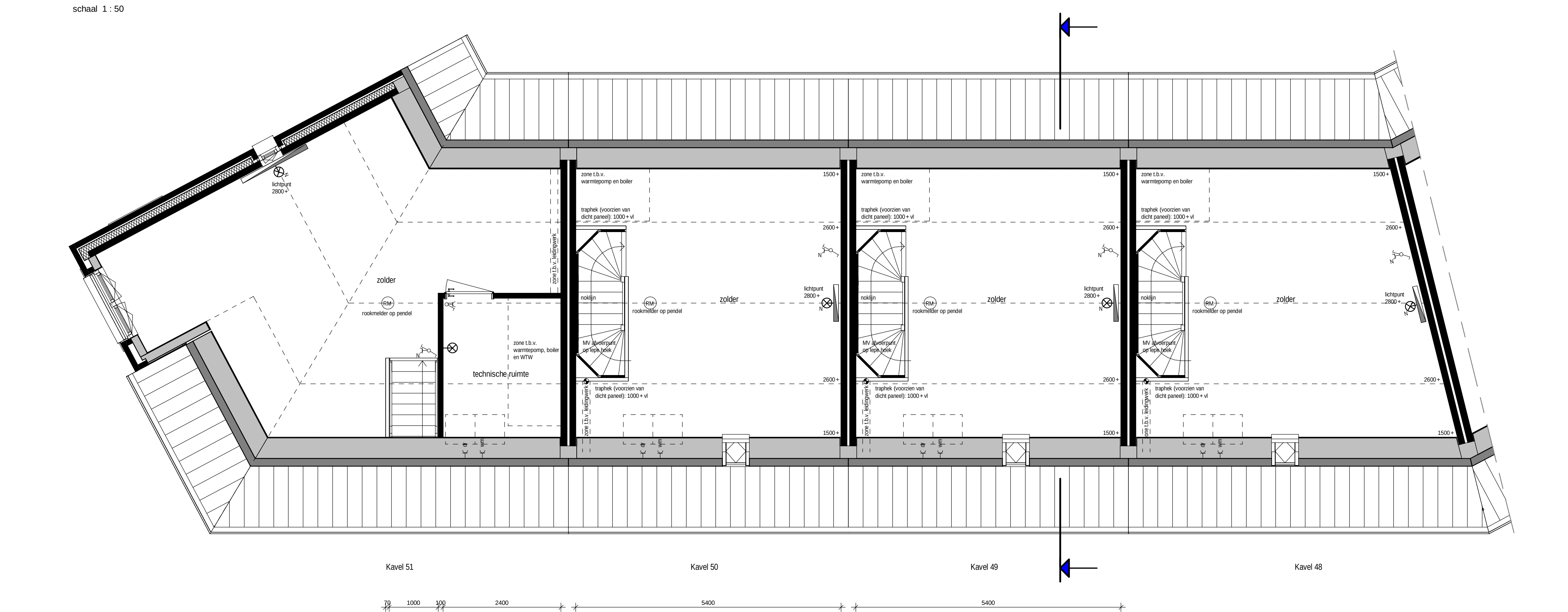
Tweede verdieping schaal 1:50
