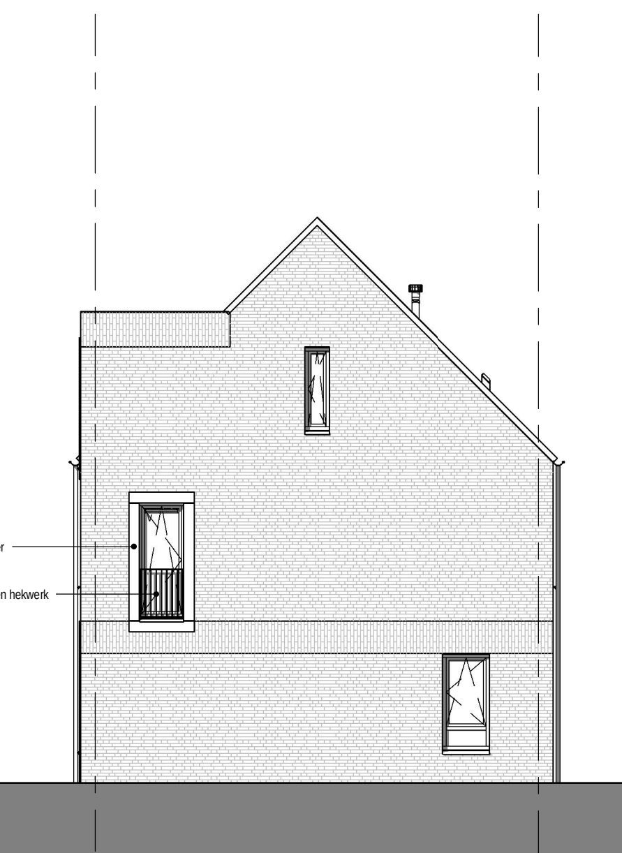
Rechter zijgevel schaal 1:100
