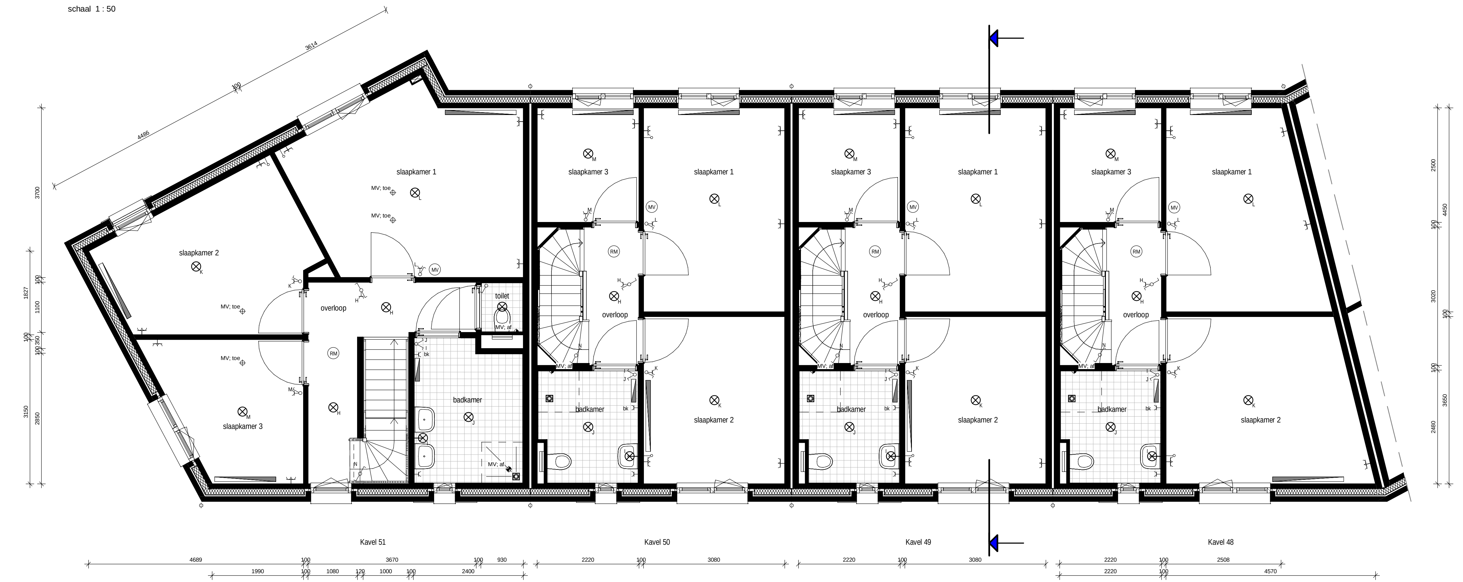
Eerste verdieping schaal 1:50
