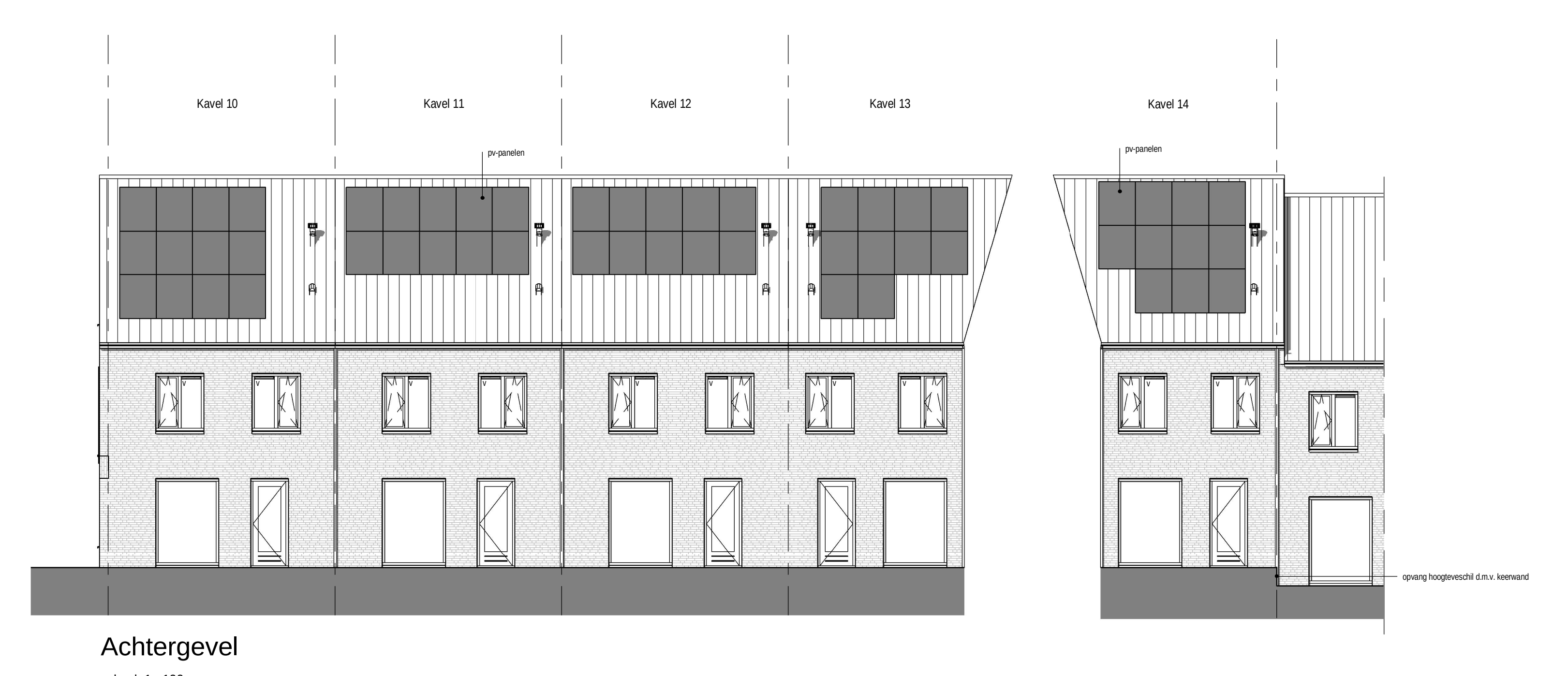
Achtergevel schaal 1:100
