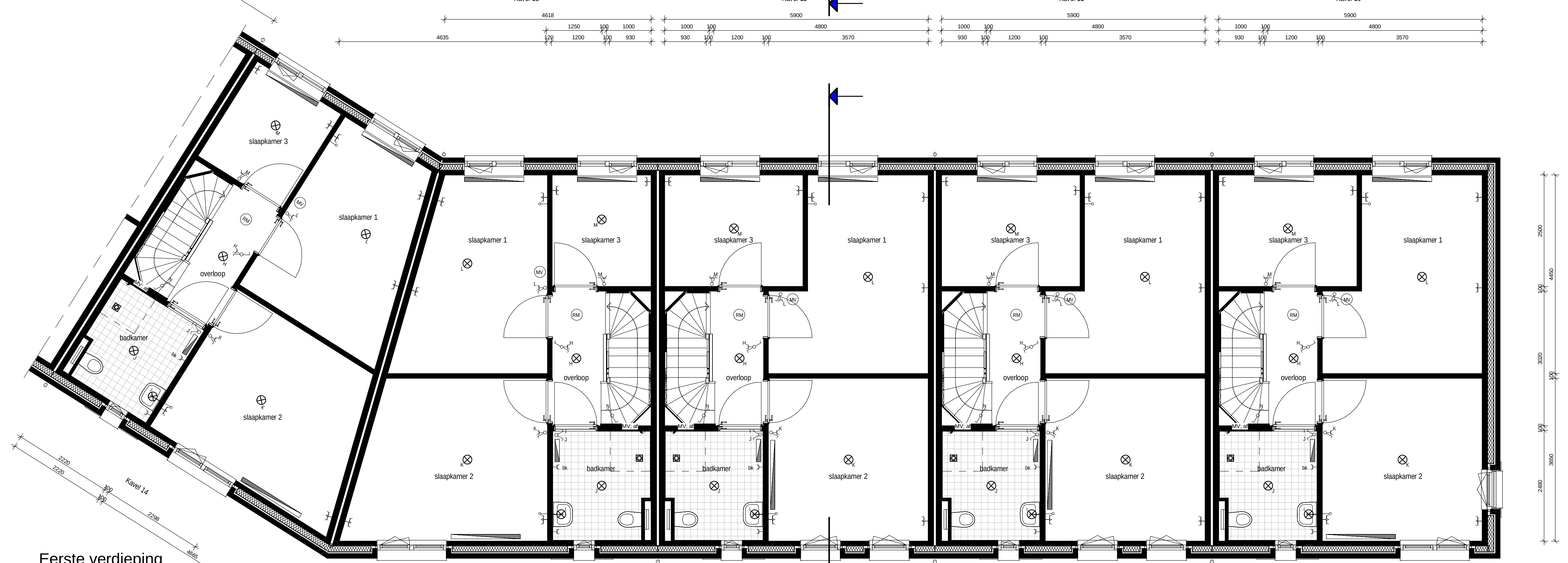
Eerste verdieping schaal 1:50
