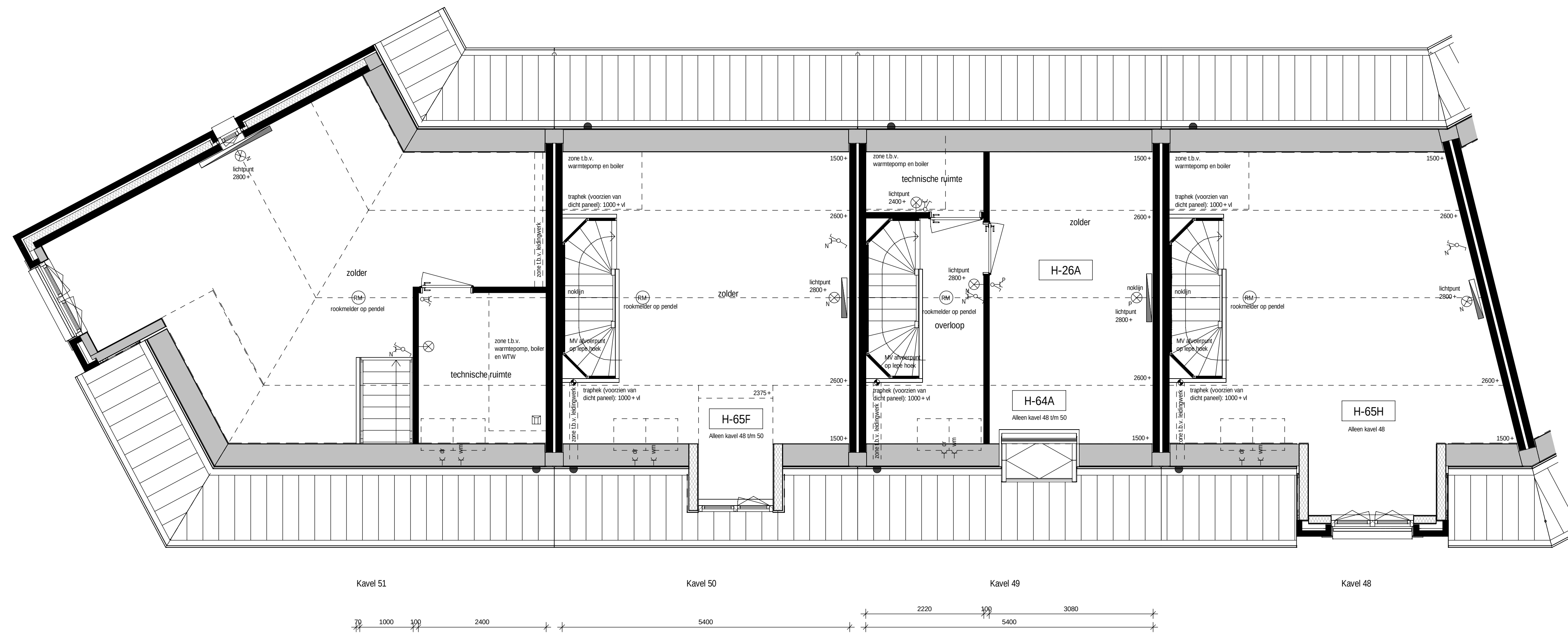
Tweede verdieping schaal 1 : 50
