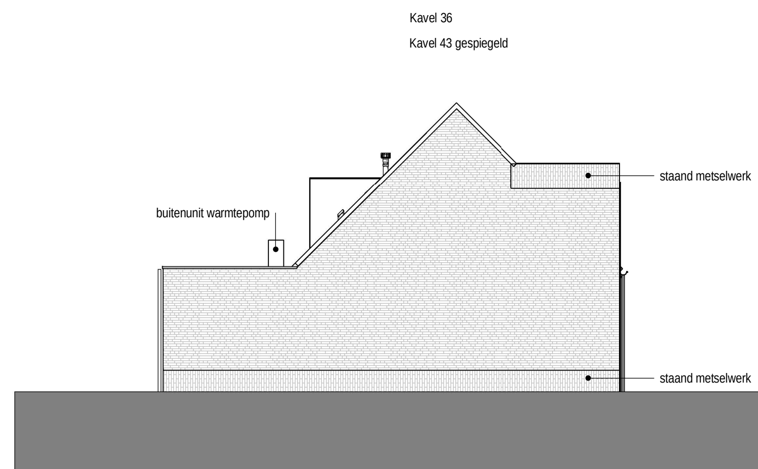
Zijgevel schaal 1 : 100
