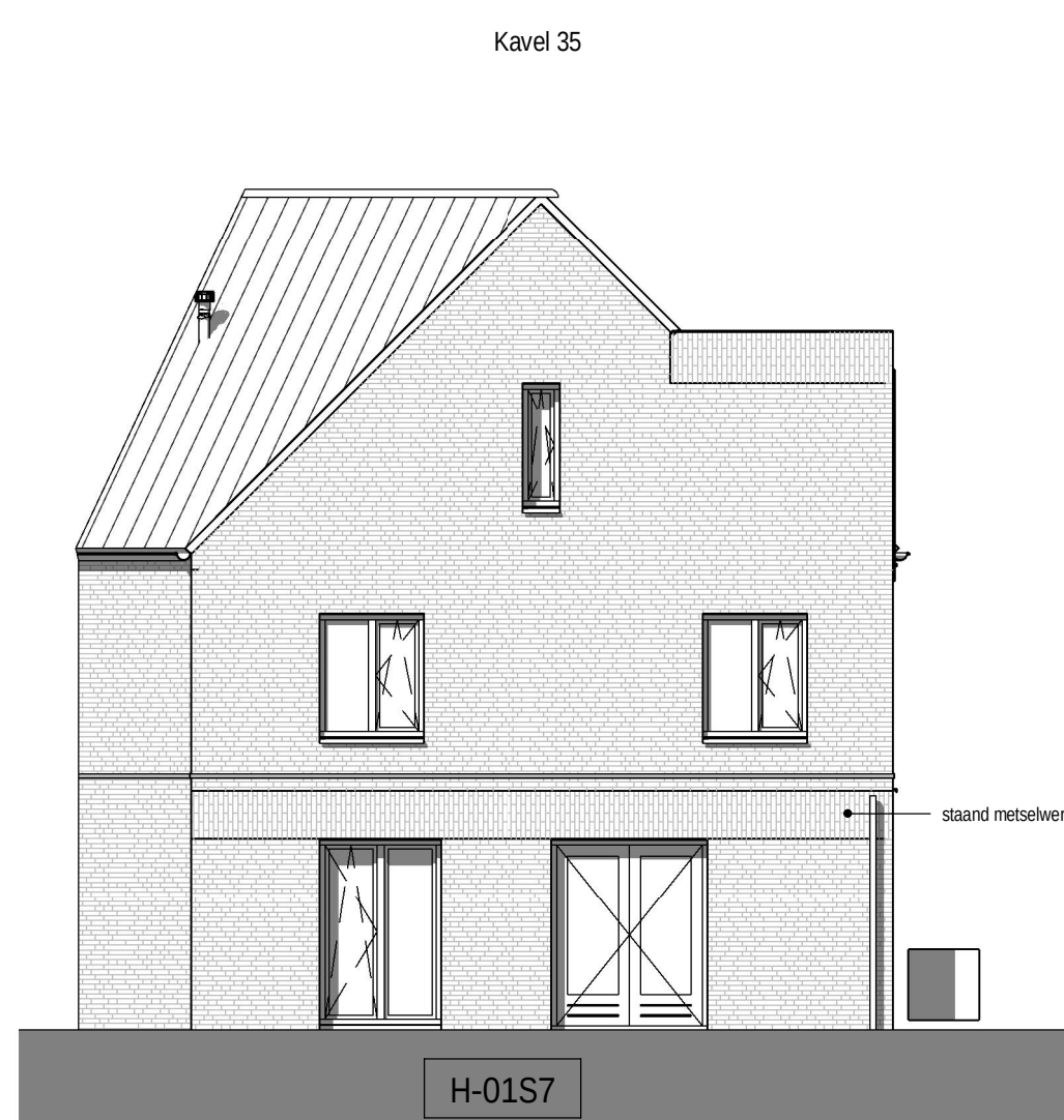
Zijgevel
