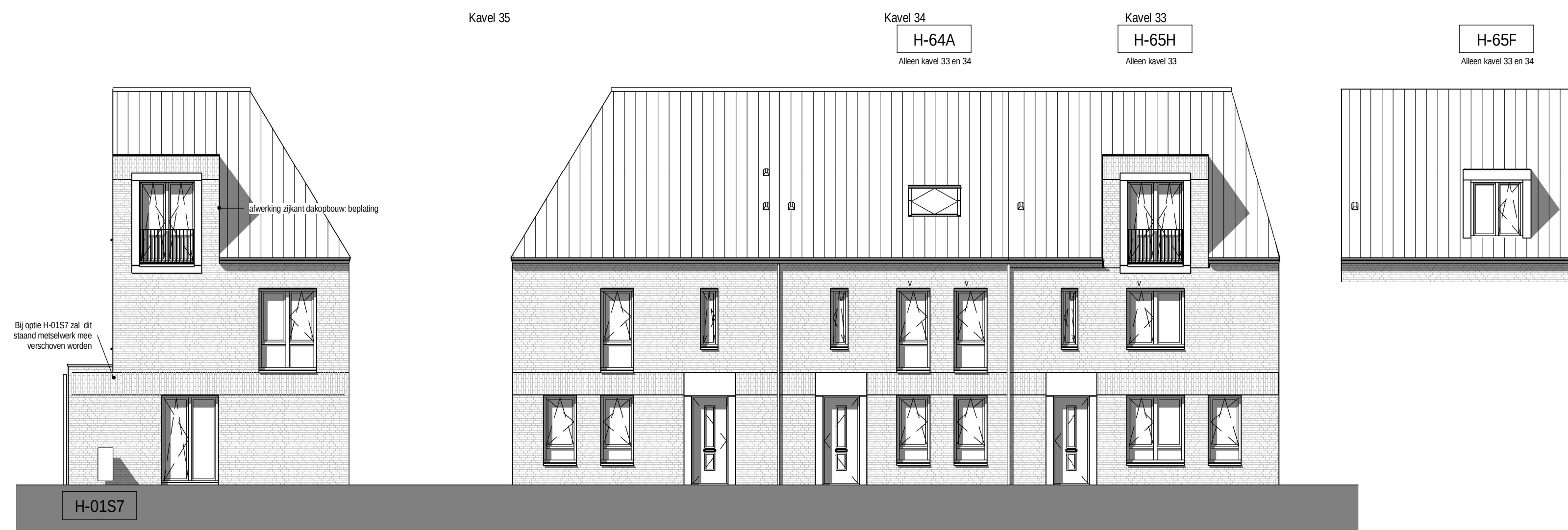
Voorgevel
