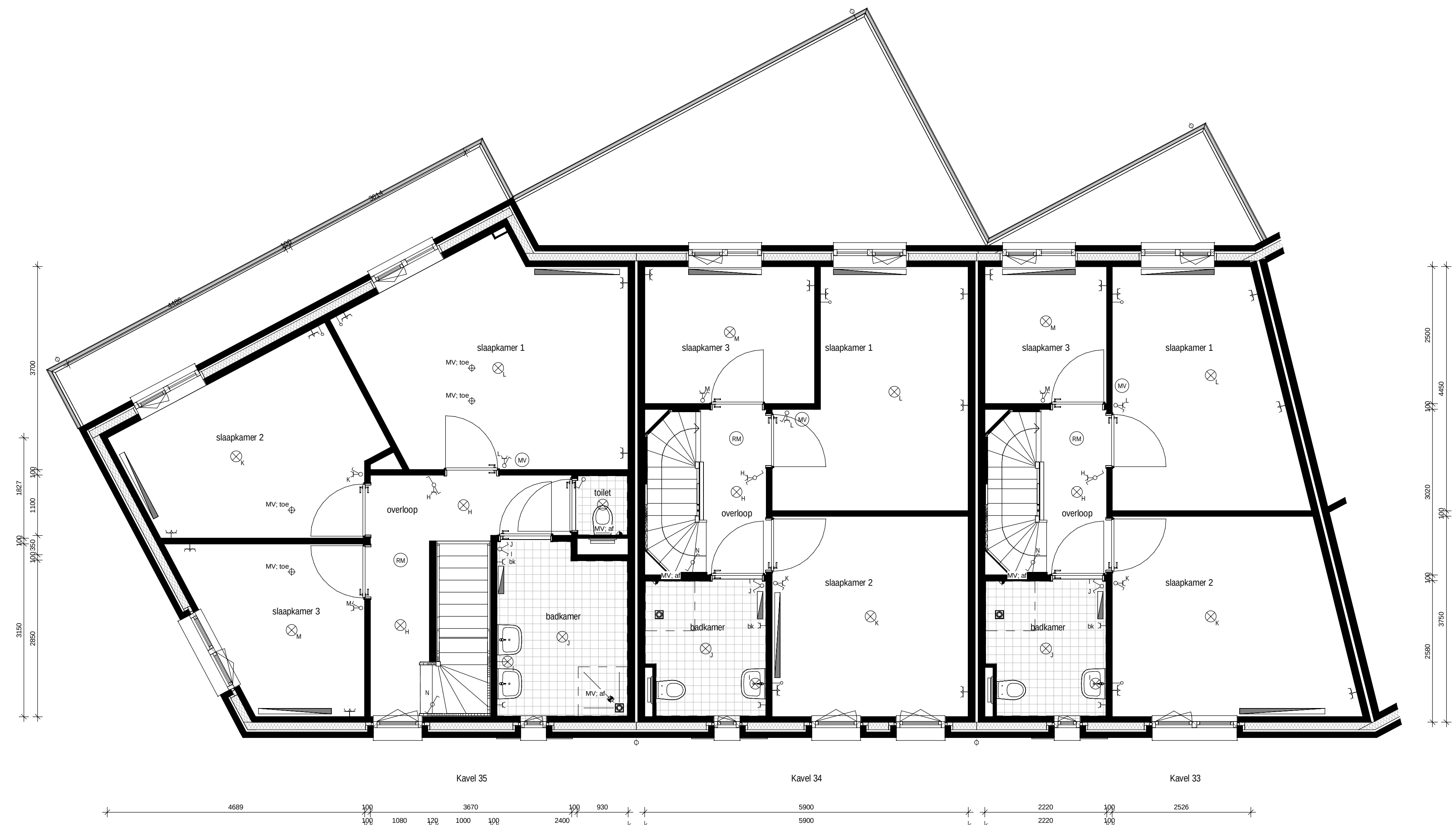
Eerste verdieping
