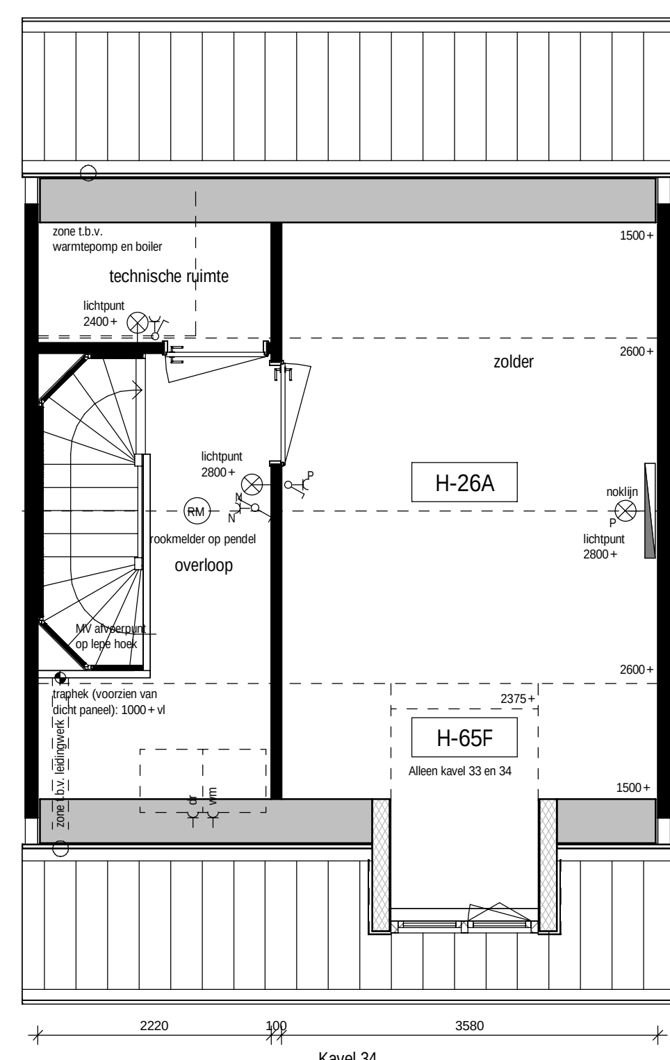
Tweede verdieping
