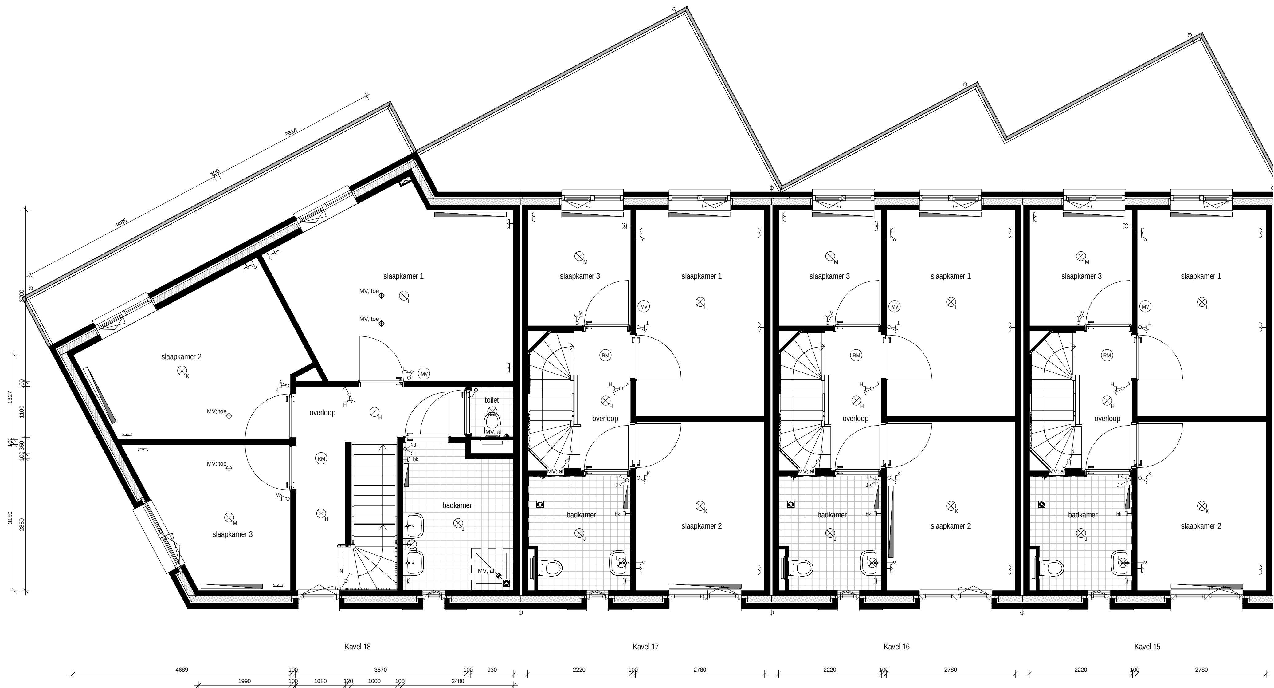
Eerste verdieping schaal 1 : 50
