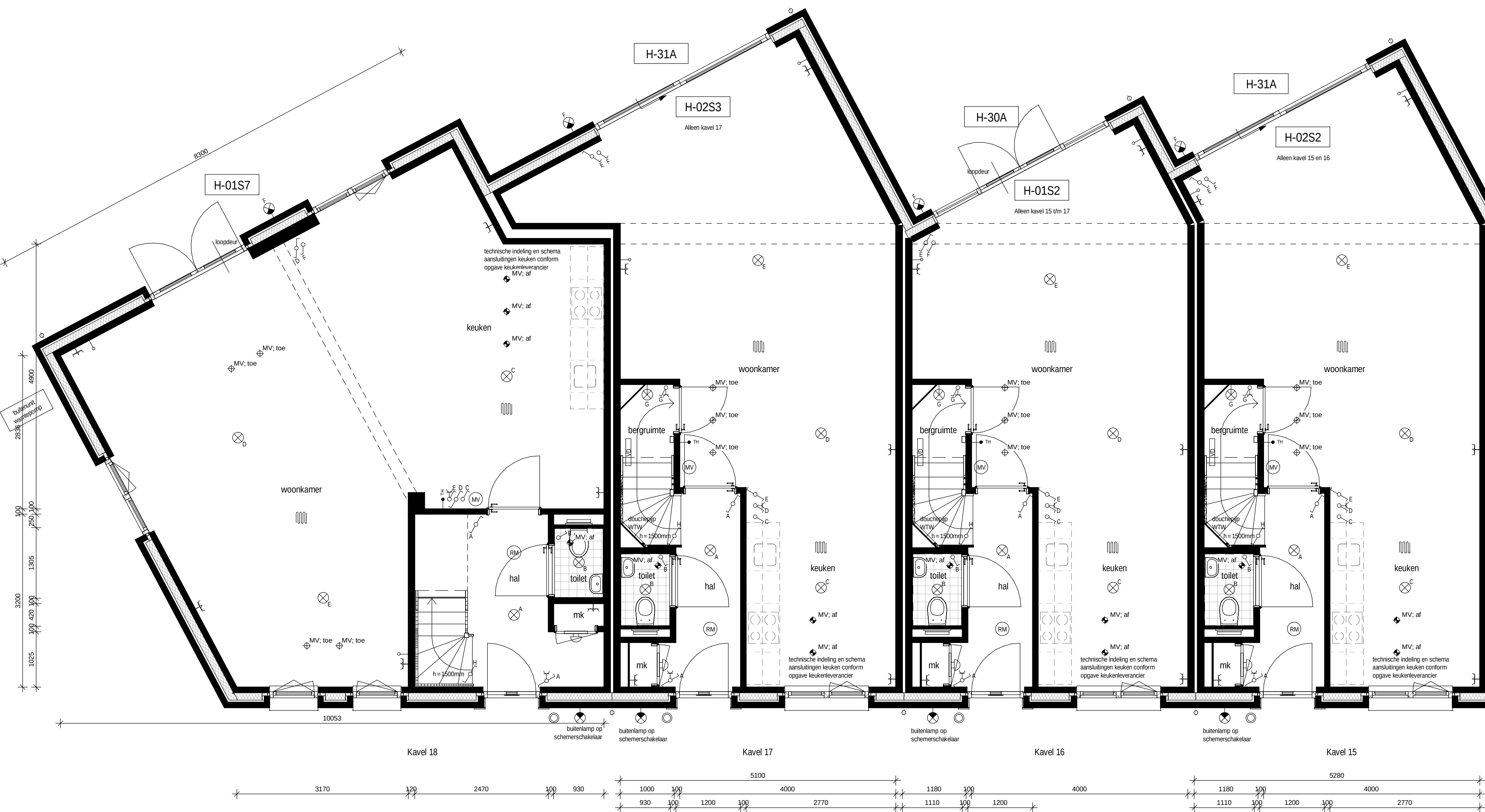
Begane grond schaal 1 : 50
