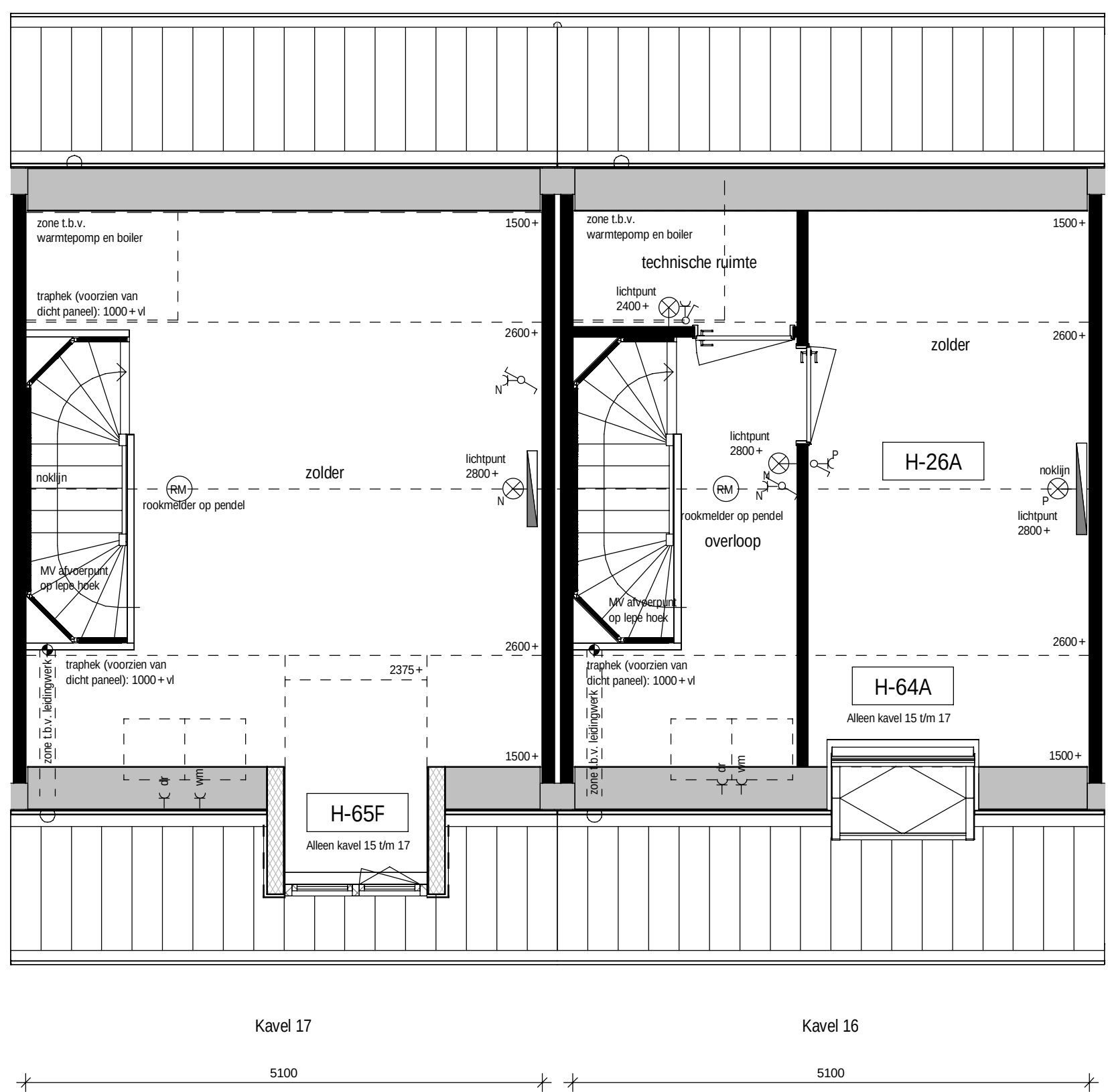
Tweede verdieping schaal 1 : 50
