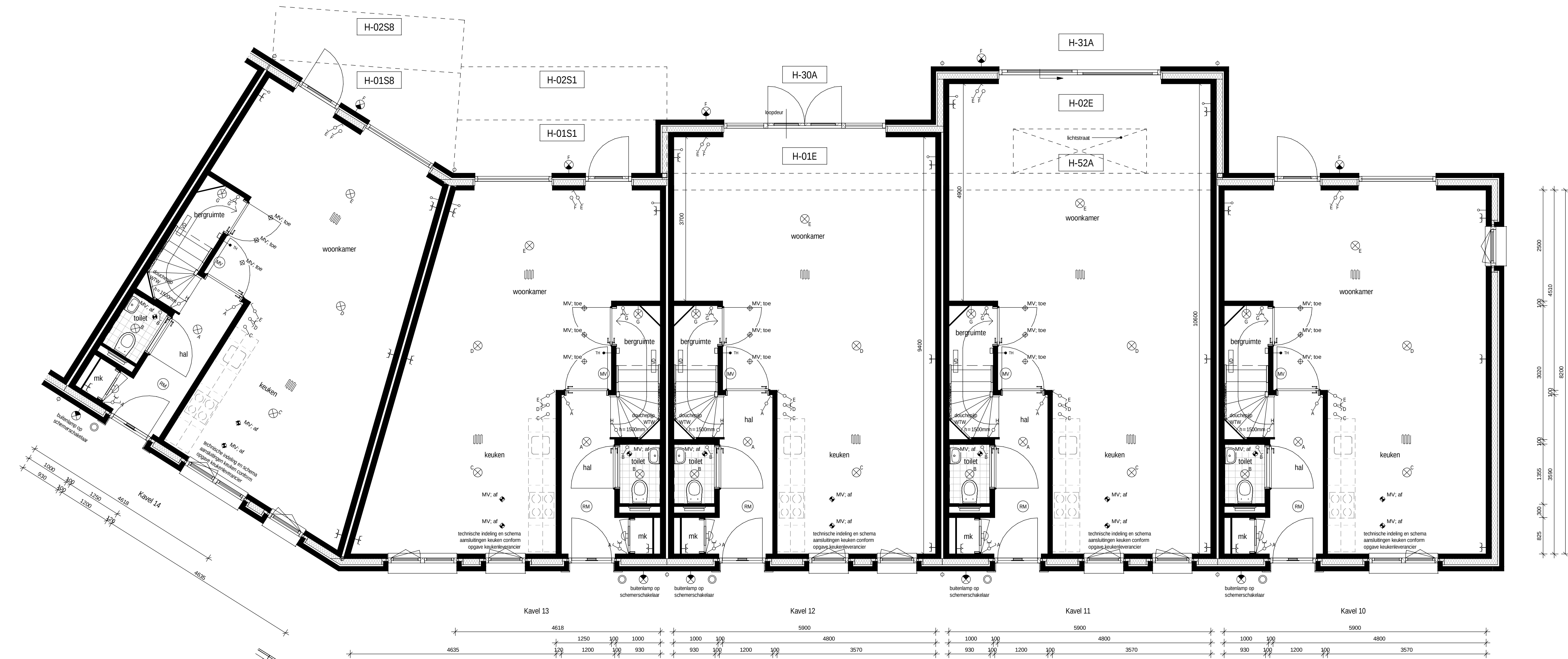
Begane grond schaal 1 : 50
